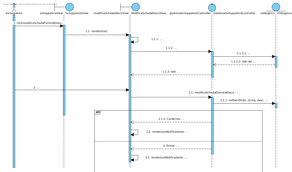
Figura 33: Sequence Diagram - Gestione Scheda del Videogioco
