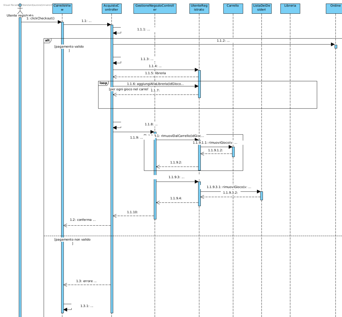
Figura 26: Sequence Diagram - Acquisto Videogioco
