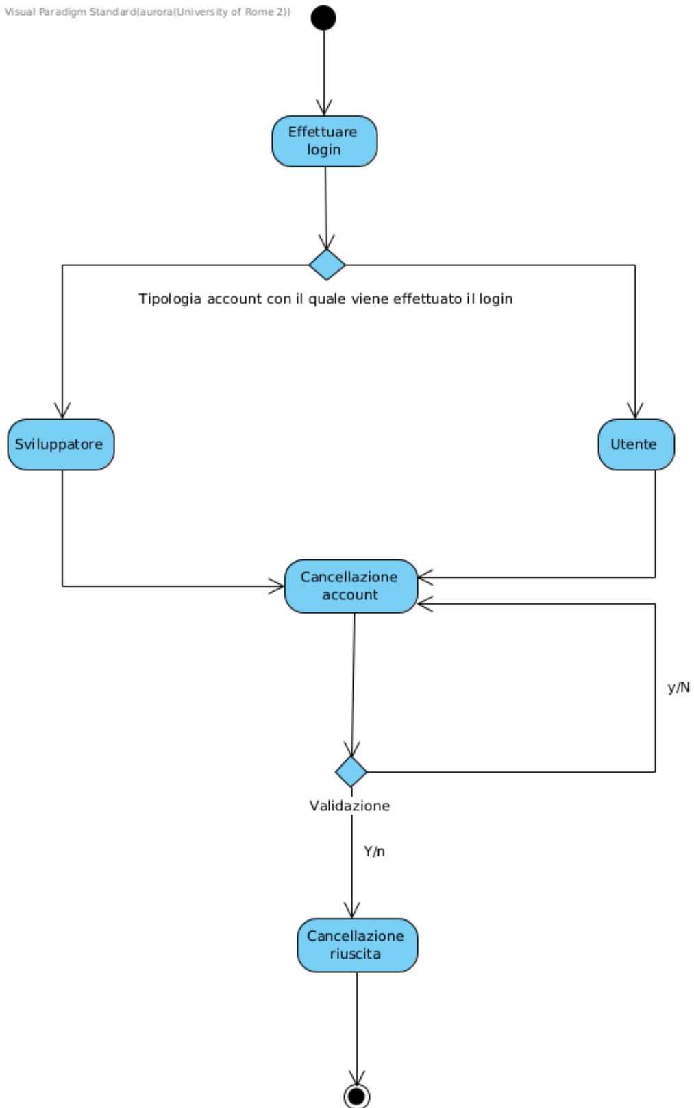
Figura 8: Activity Diagram - Cancellazione account
