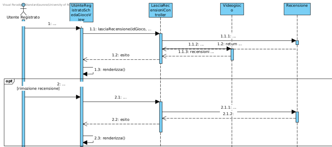
Figura 29: Sequence Diagram - Recensione Videogioco
