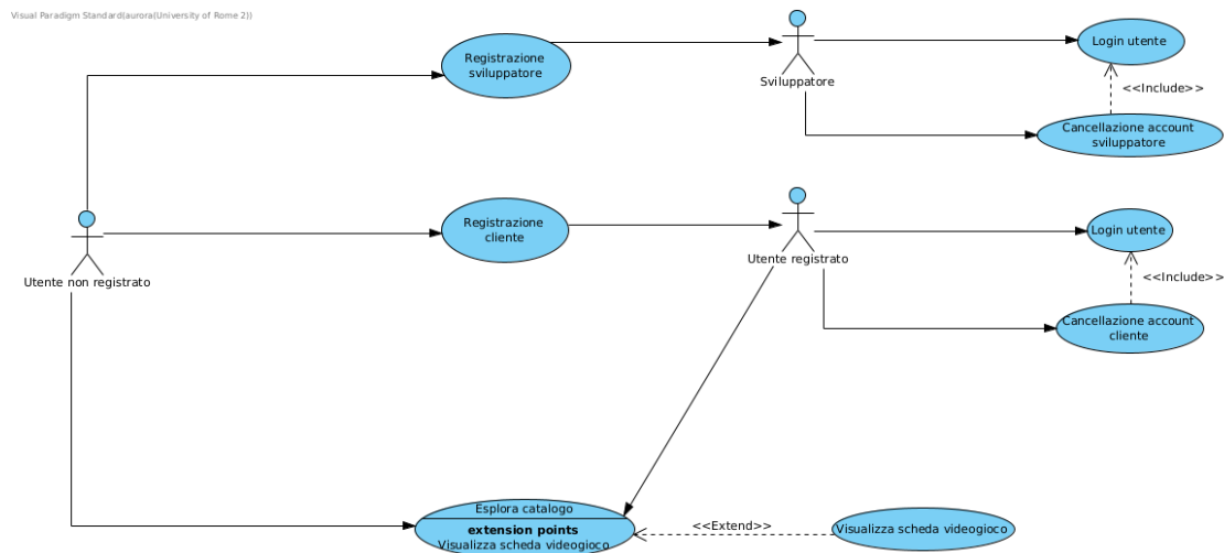
Figura 1: Use case Diagram Utente non registrato
