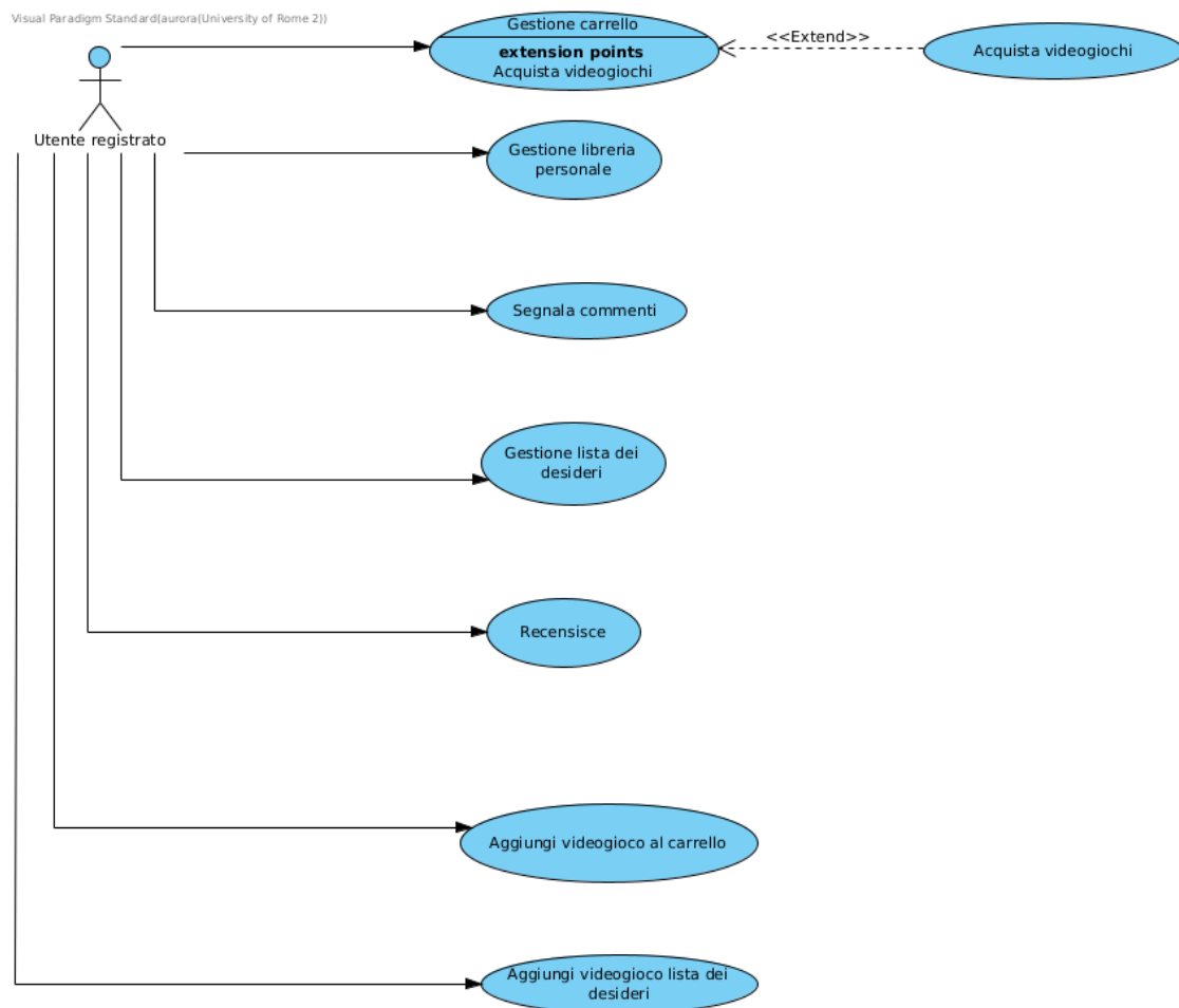
Figura 2: Use case Diagram Utente registrato
