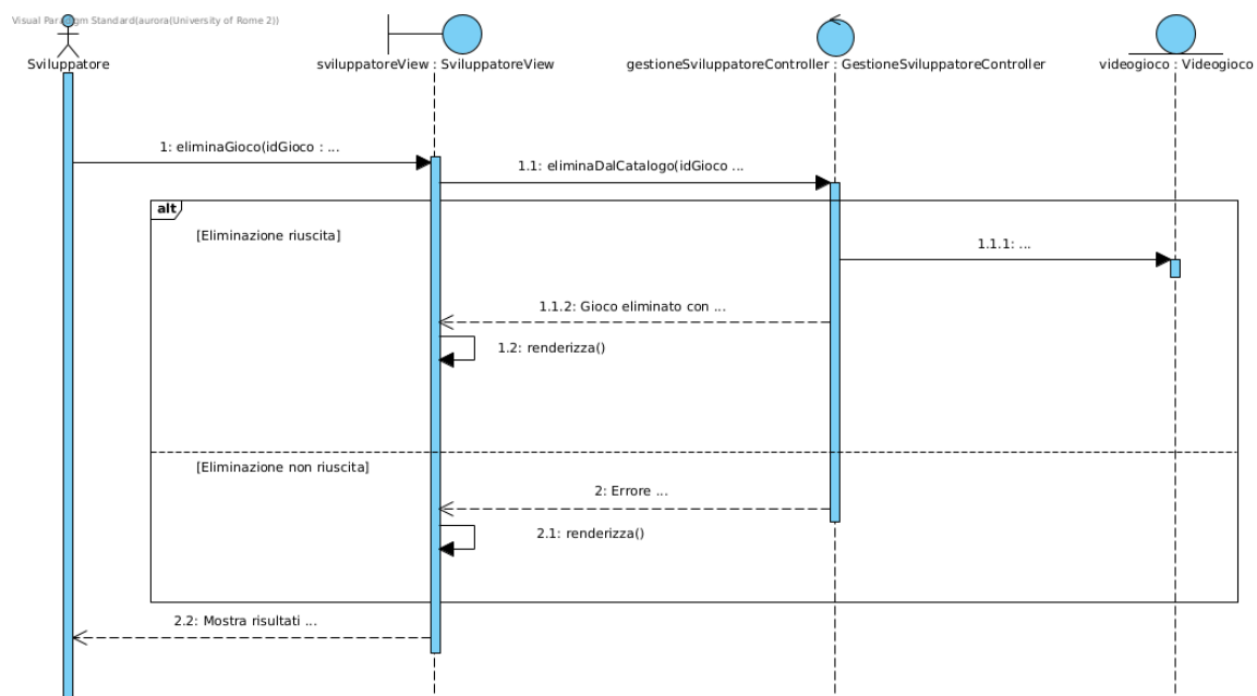
Figura 34: Sequence Diagram - Cancellazione Videogioco
