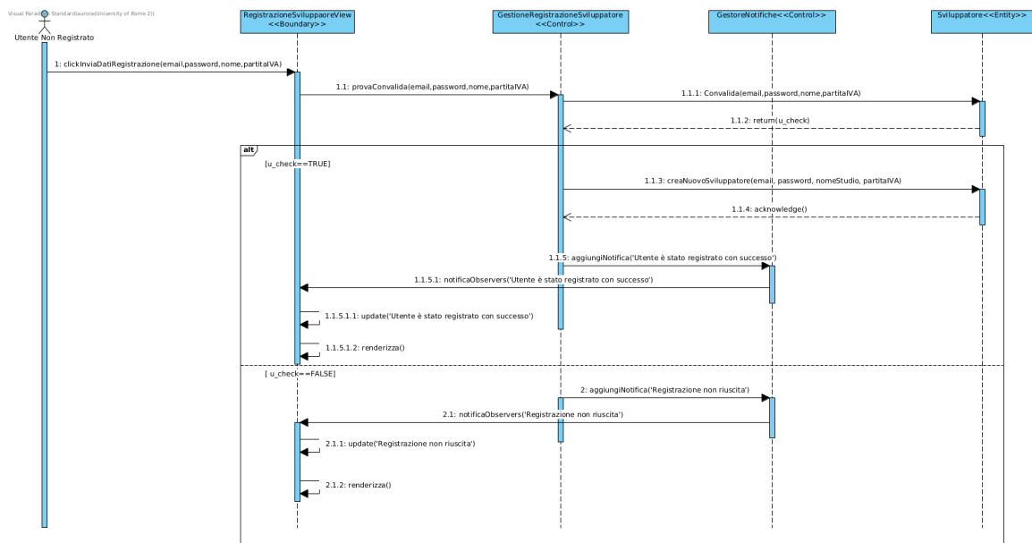
Figura 22: Sequence Diagram - Registrazione Sviluppatore
