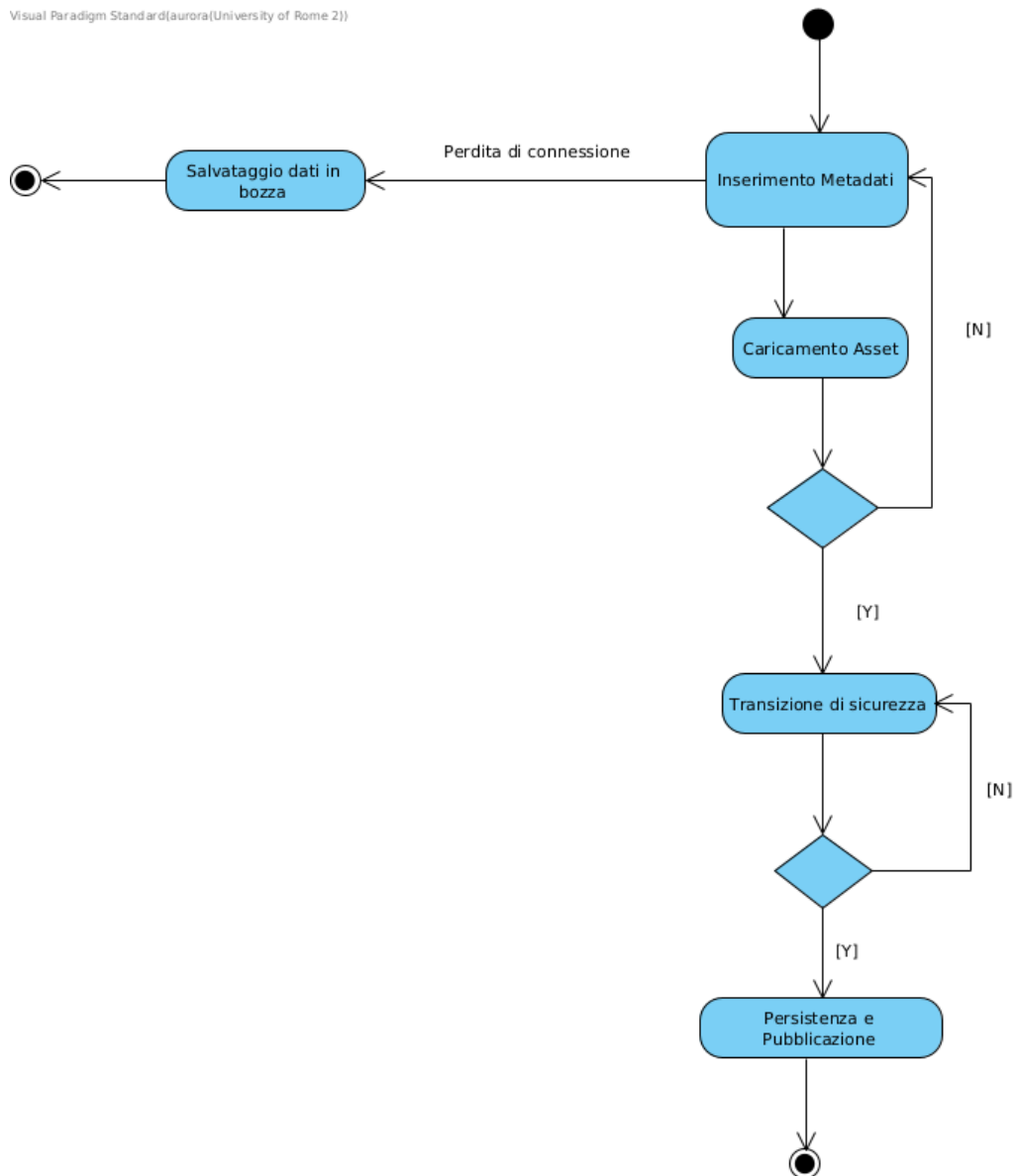
Figura 14: Activity Diagram - Upload videogioco
