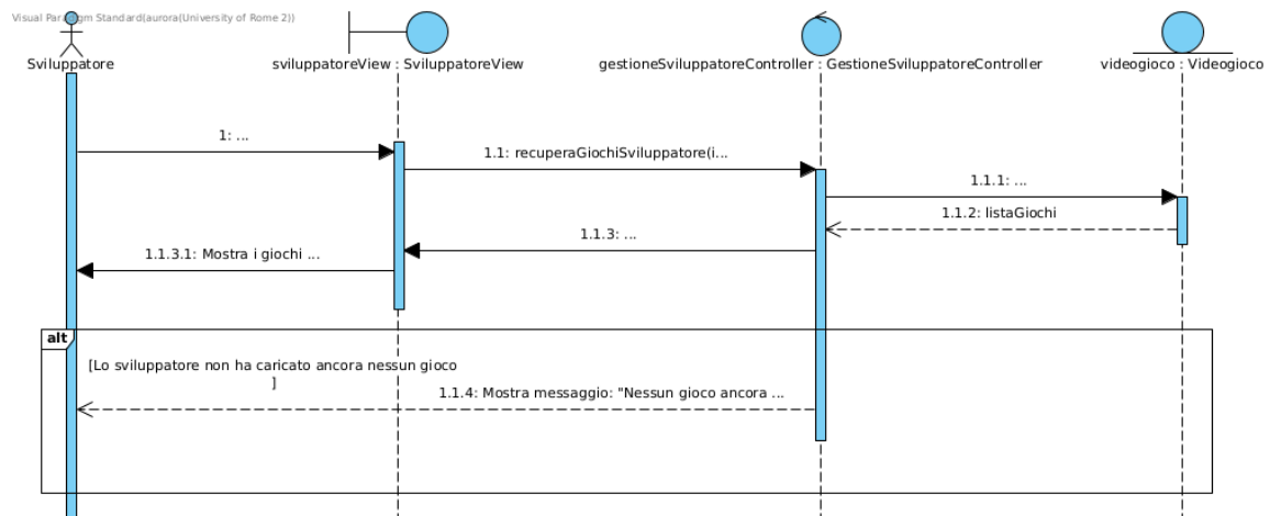
Figura 35: Sequence Diagram - Visualizzazione Giochi Sviluppati
