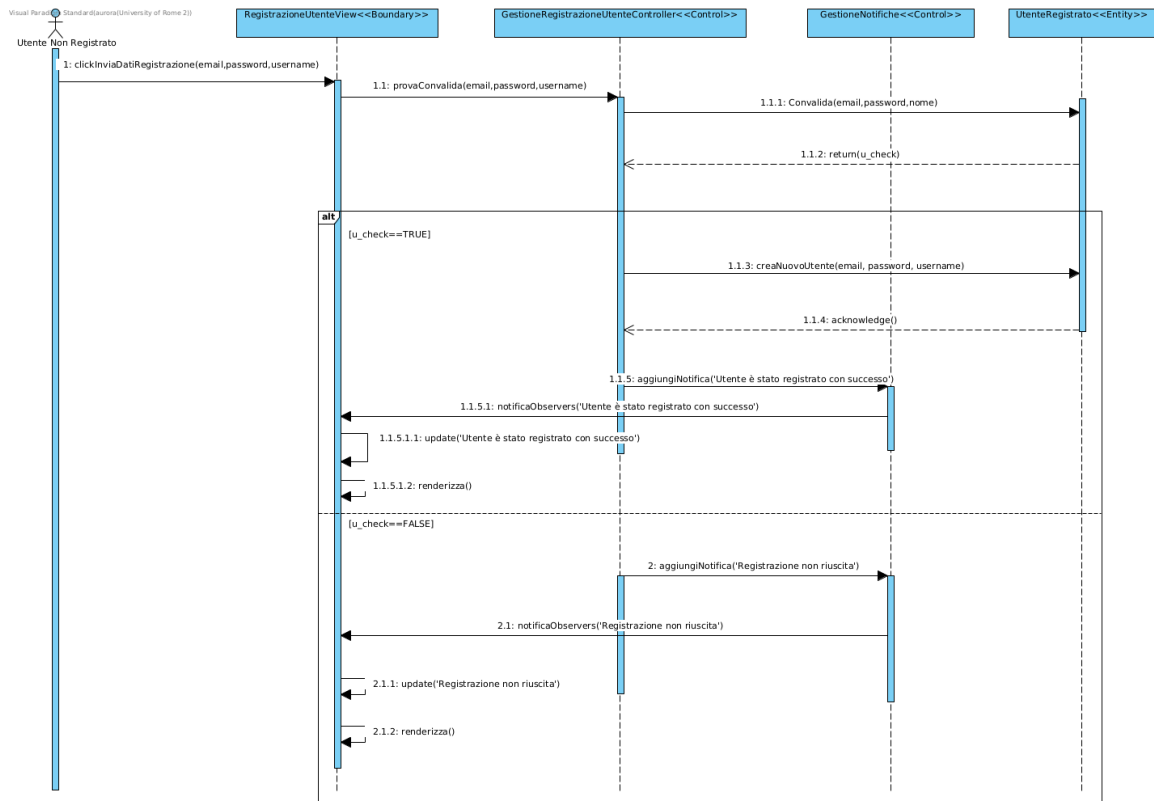
Figura 21: Sequence Diagram - Registrazione Utente
