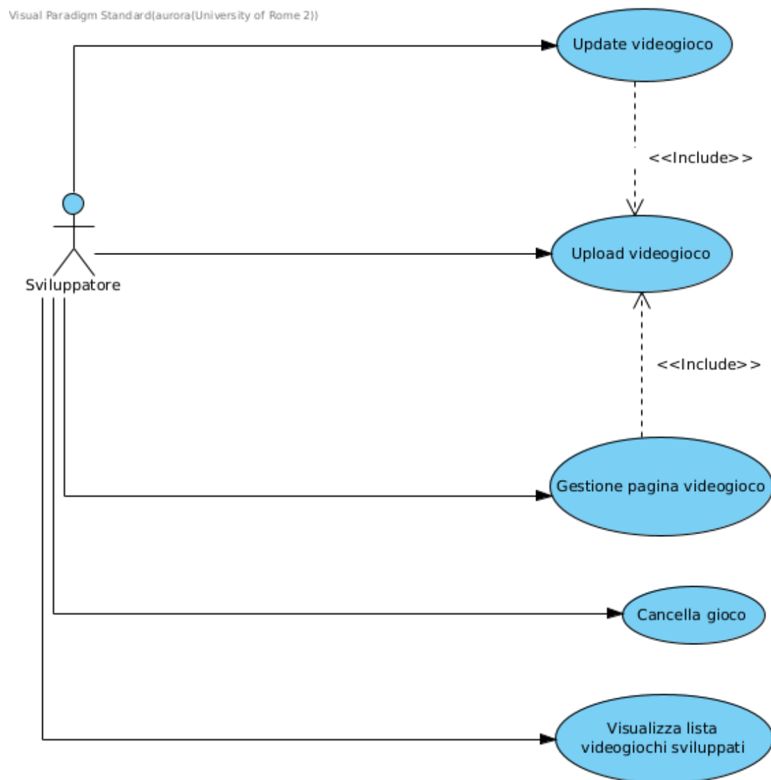
Figura 3: Use case Diagram Sviluppatore
