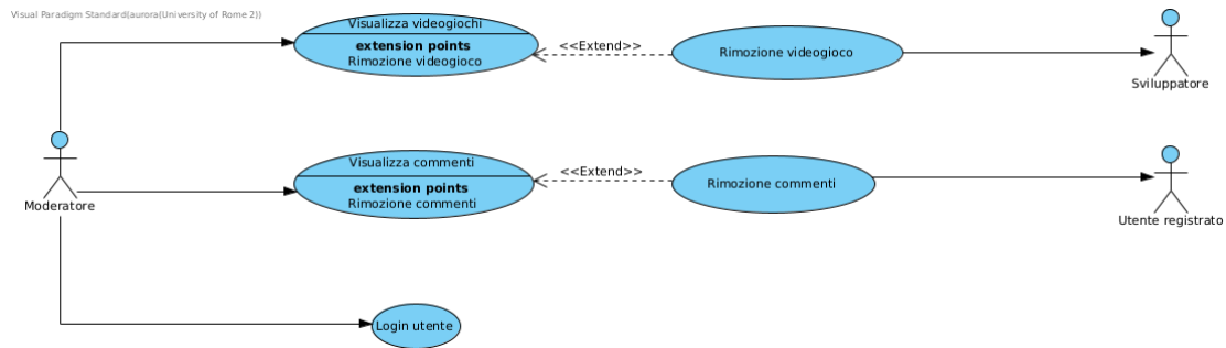
Figura 4: Use case Diagram Moderatore
