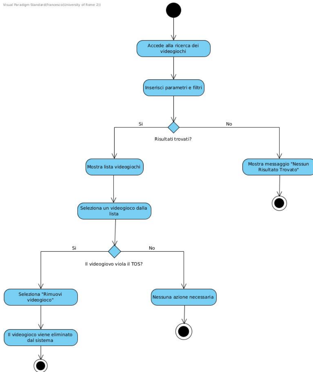
Figura 18: Activity Diagram - Gestione videogiochi
