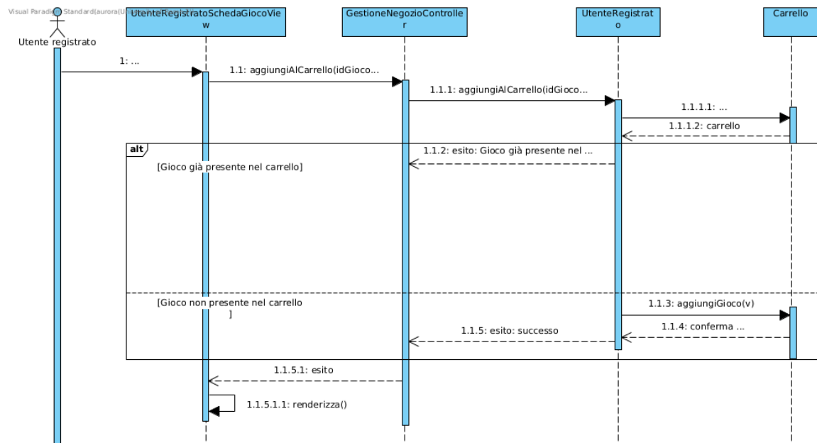
Figura 25: Sequence Diagram - Aggiunta di un videogioco al carrello
