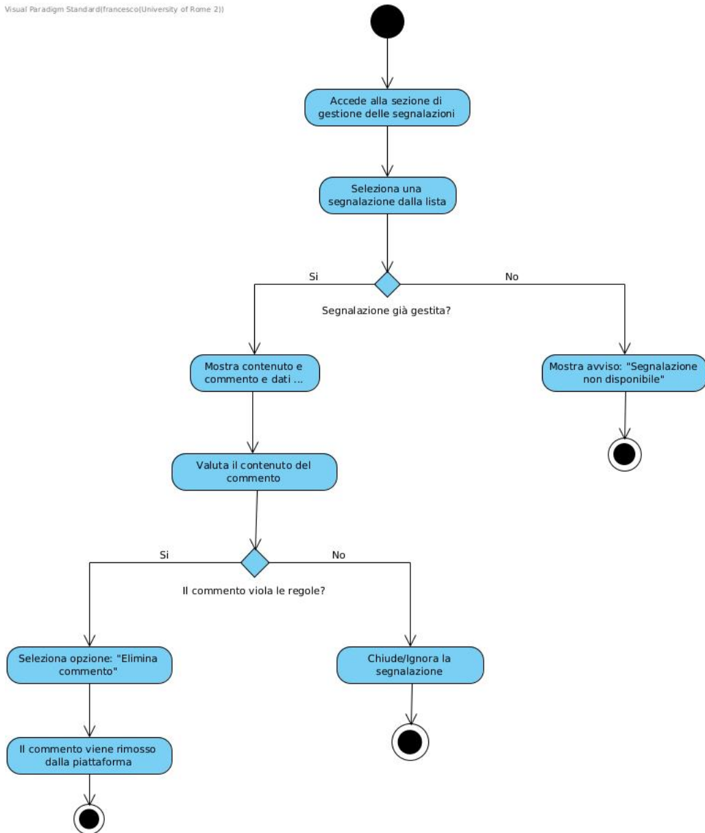
Figura 19: Activity Diagram - Gestione commenti
