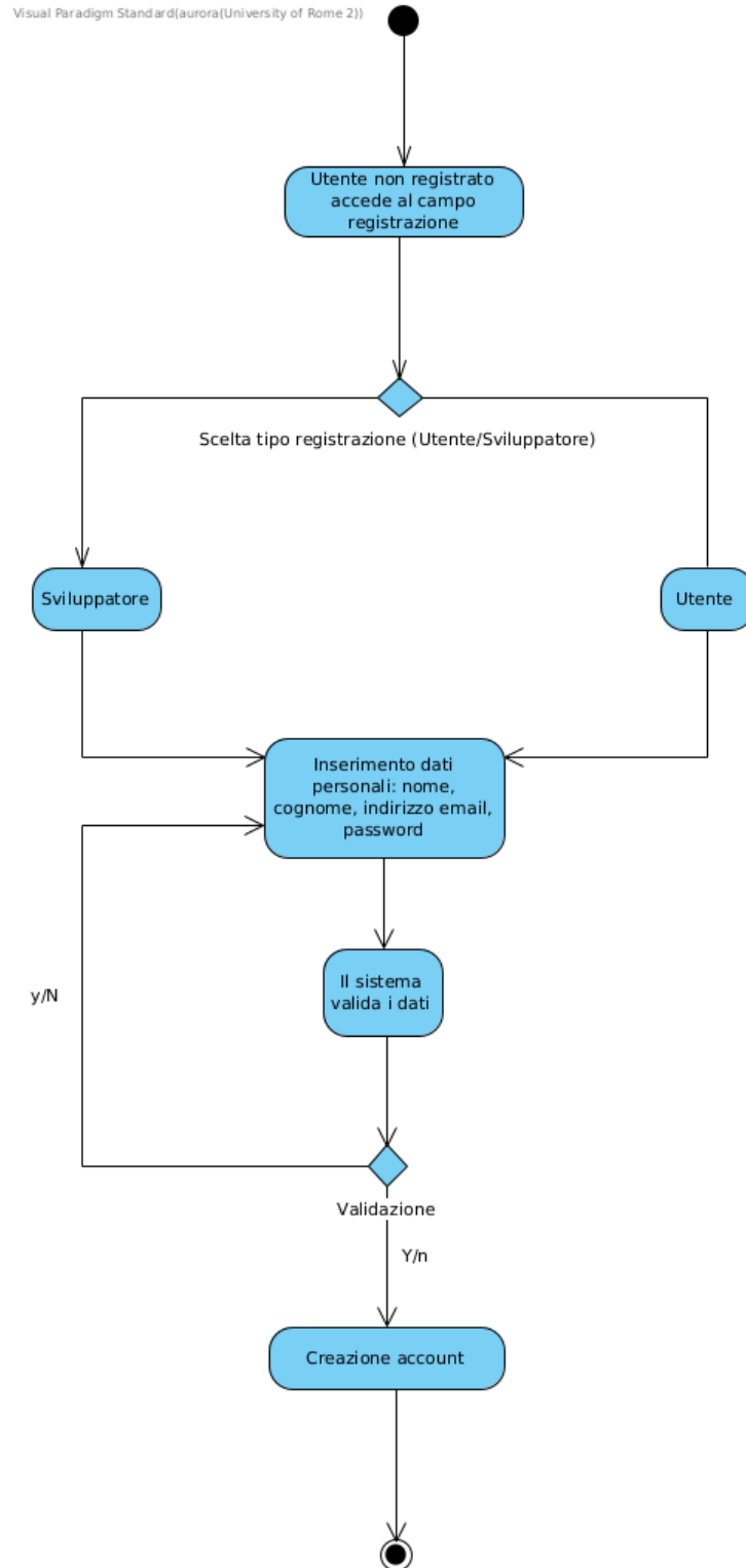
Figura 5: Activity Diagram - Registrazione
