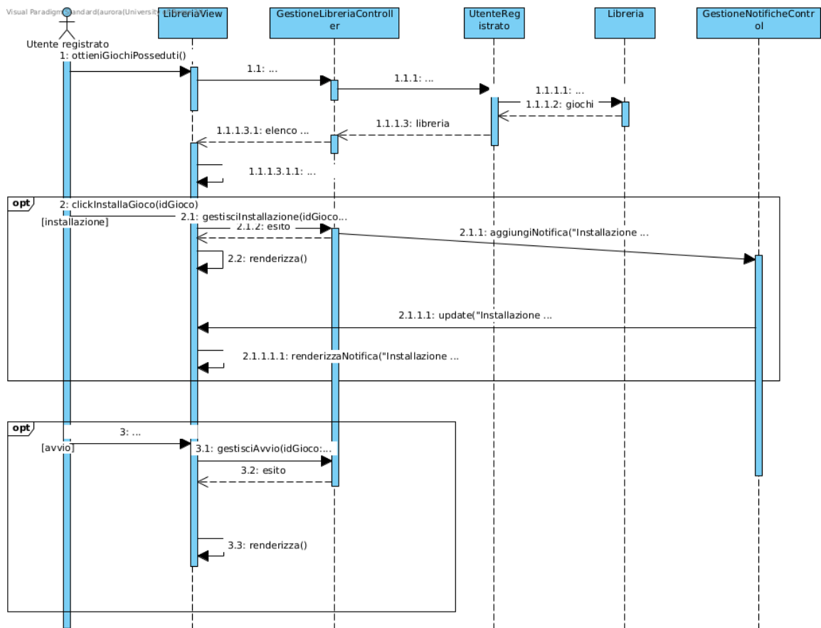
Figura 27: Sequence Diagram - Gestione Libreria Personale
