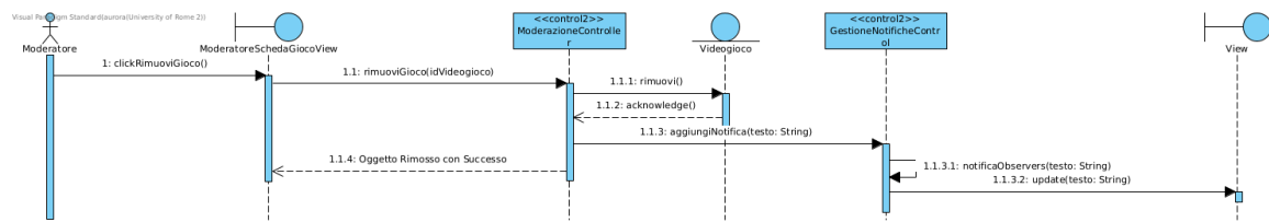
Figura 38: Sequence Diagram - Eliminazione Videogioco da parte del Moderatore
