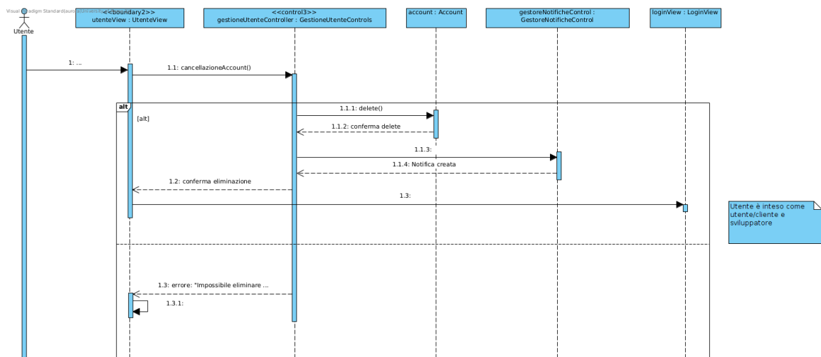
Figura 24: Sequence Diagram - Cancellazione Account
