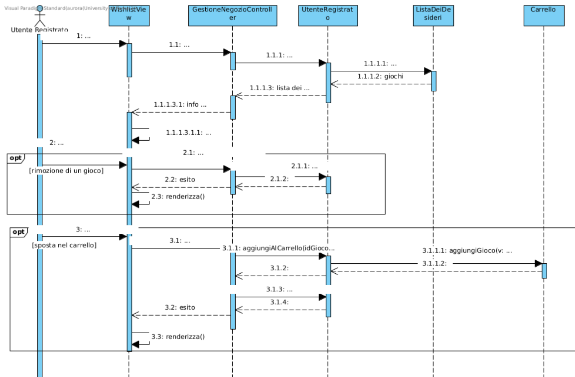
Figura 28: Sequence Diagram - Gestione Lista dei Desideri
