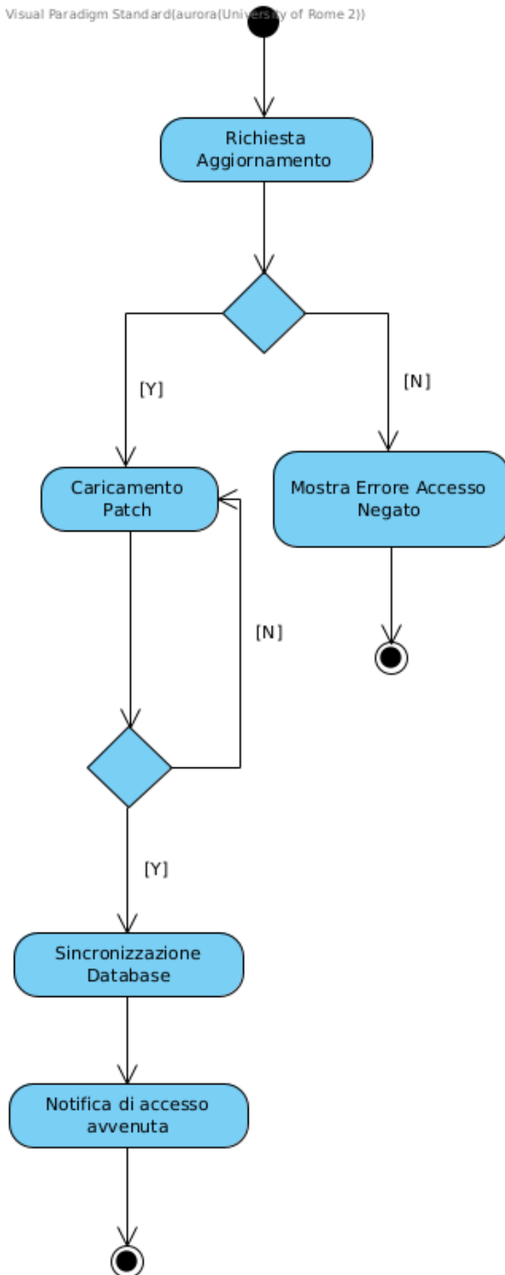
Figura 15: Activity Diagram - Aggiornamento videogioco
