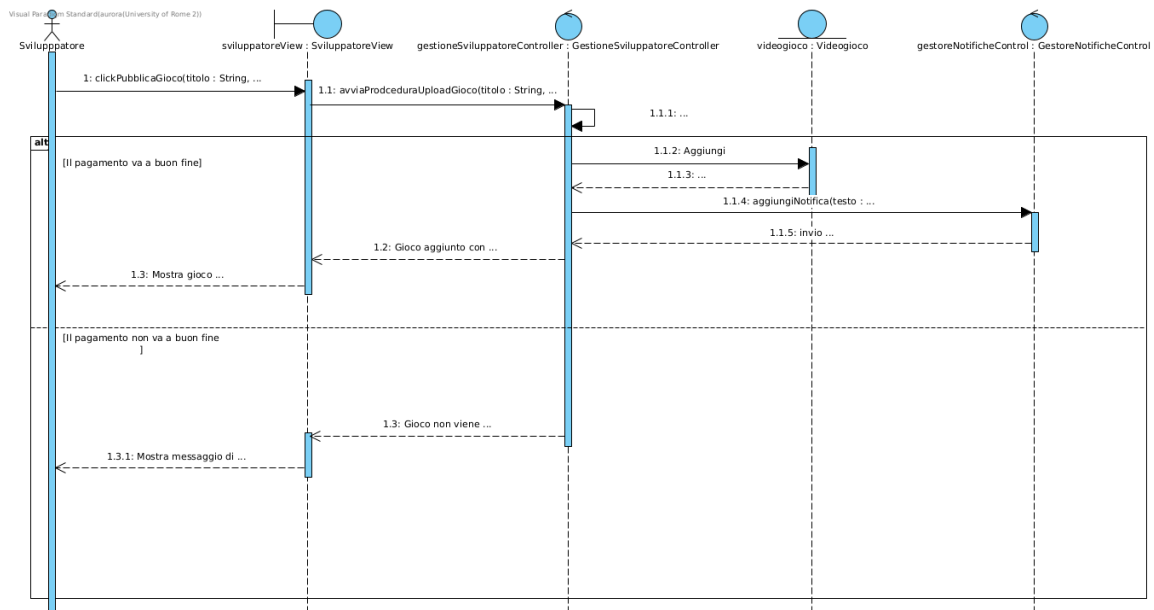
Figura 31: Sequence Diagram - Pubblicazione Videogioco
