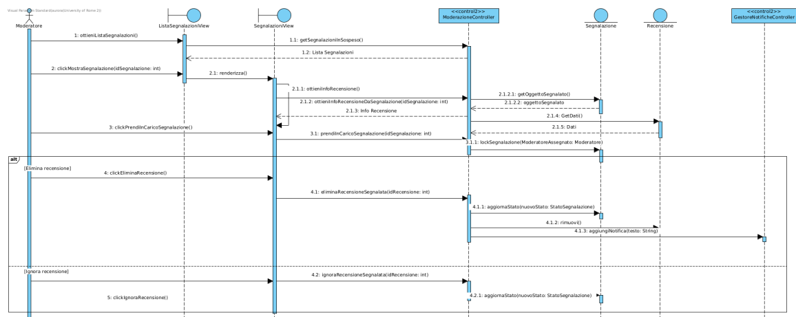
Figura 37: Sequence Diagram - Elimina o Ignora Recensione
