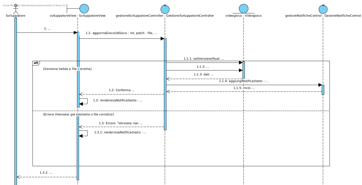
Figura 32: Sequence Diagram - Aggiornamento Videogioco
