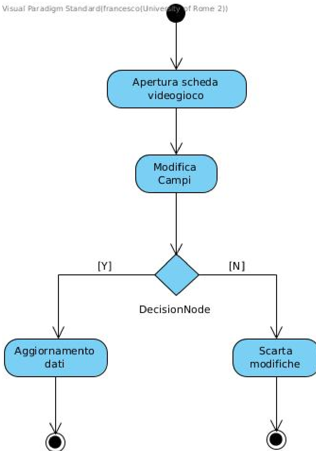
Figura 16: Activity Diagram - Gestione scheda videogioco
