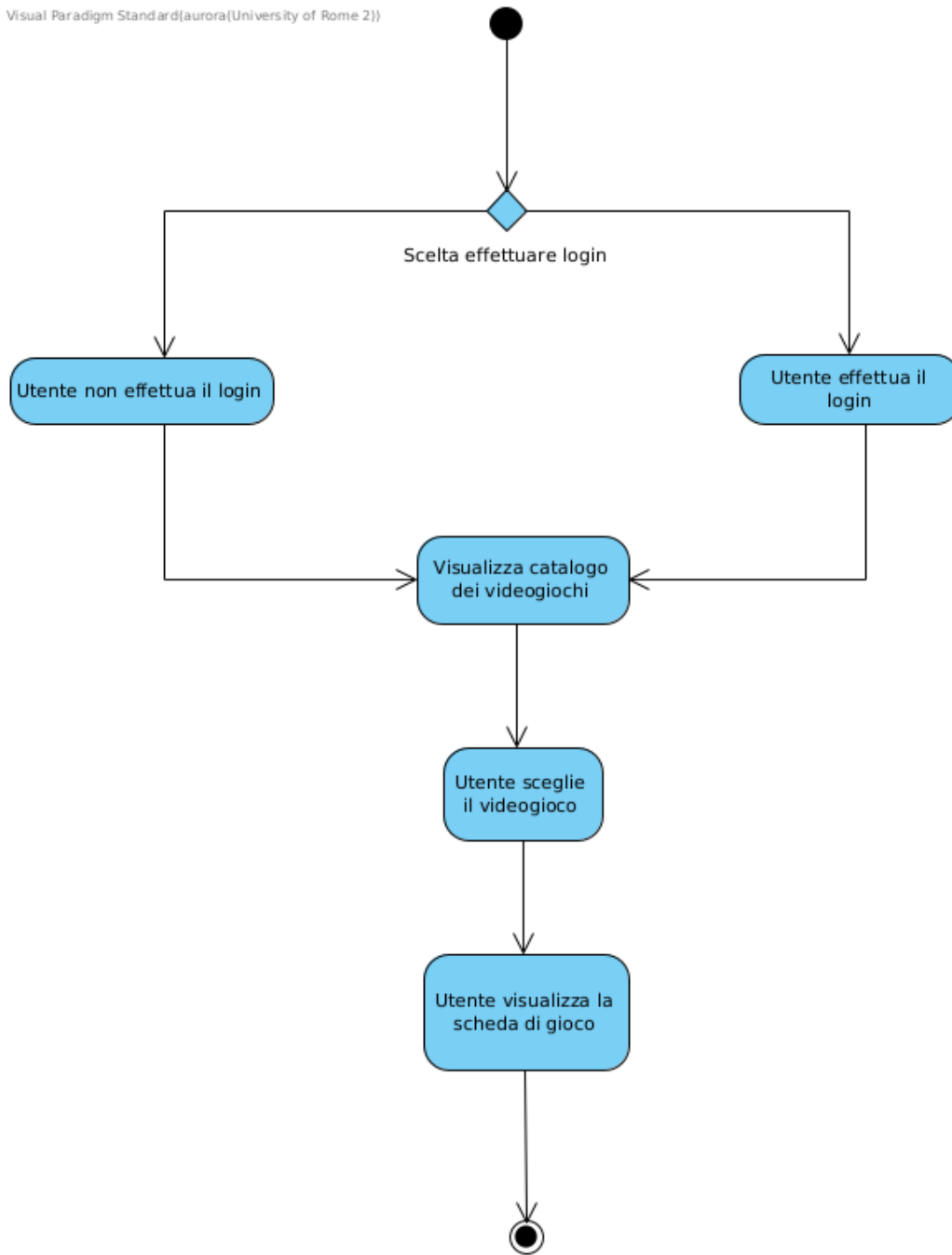
Figura 7: Activity Diagram - Esplorazione catalogo
