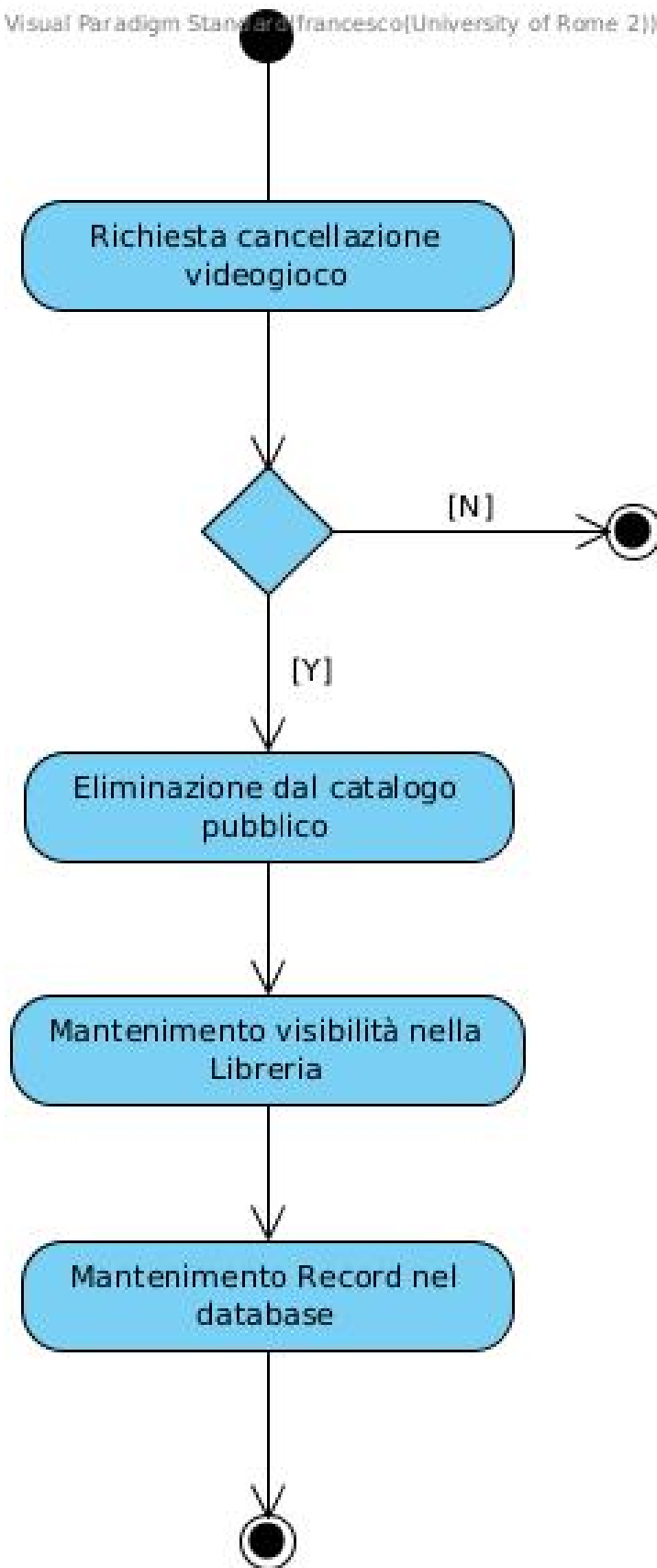
Figura 17: Activity Diagram - Cancellazione videogioco
