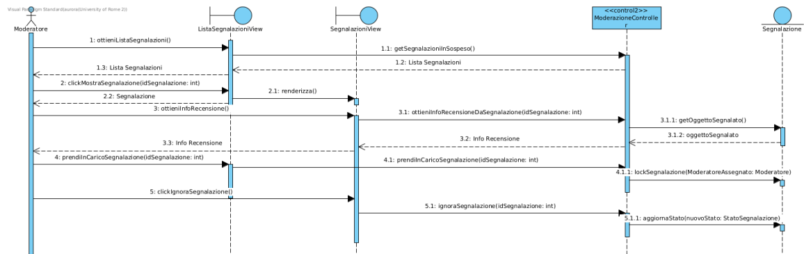
Figura 36: Sequence Diagram - Ignora Segnalazione
