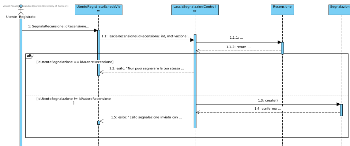
Figura 30: Sequence Diagram - Segnalazione Recensione
